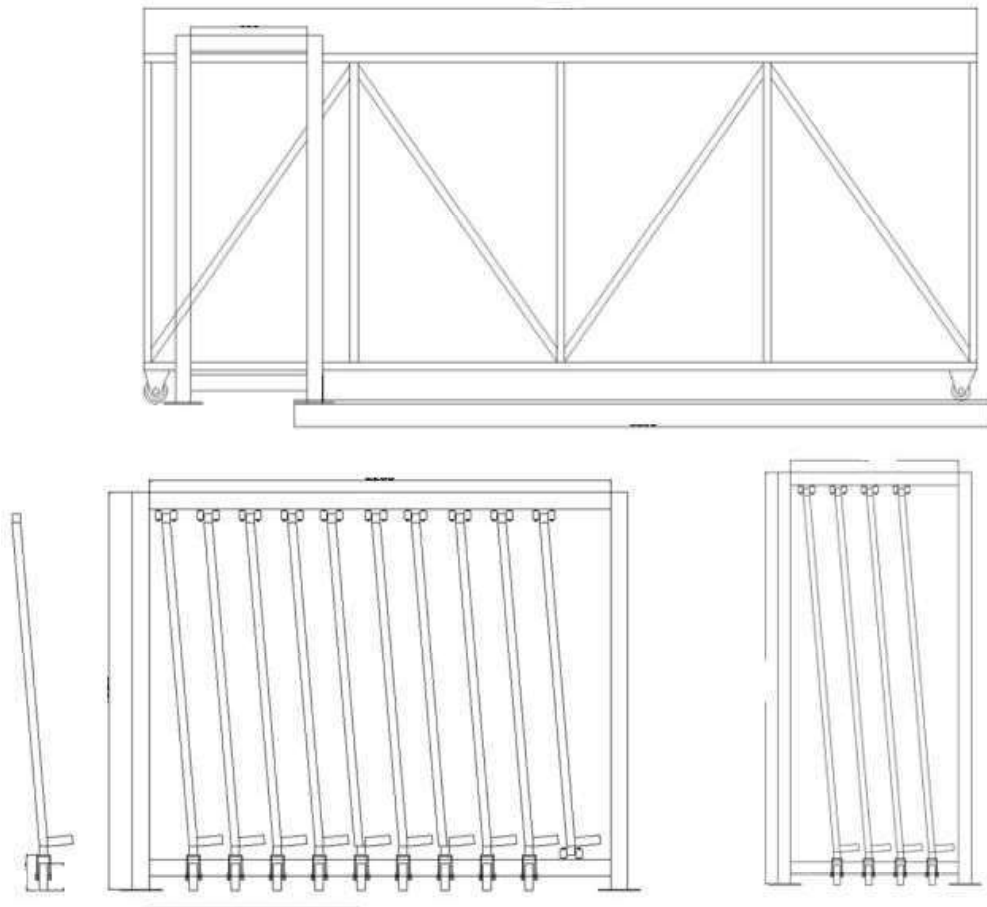
Εικόνα 1 Ενδεικτική γεωμετρία των δύο τύπων συστημάτων αποθήκευσης
